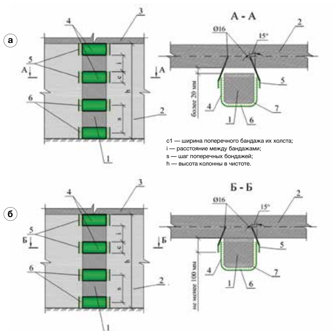
Рис. Г.4.11. Схема усиления колон-пилястр: а) с зазором более 20 мм; б) без зазора.
