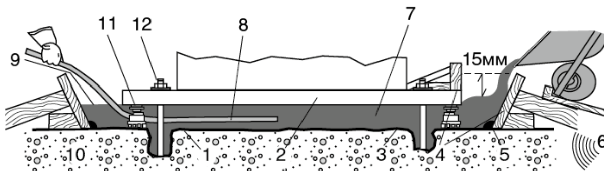
Рисунок 1: Схема применения MasterFlow 928 для высокоточной цементации оборудования
